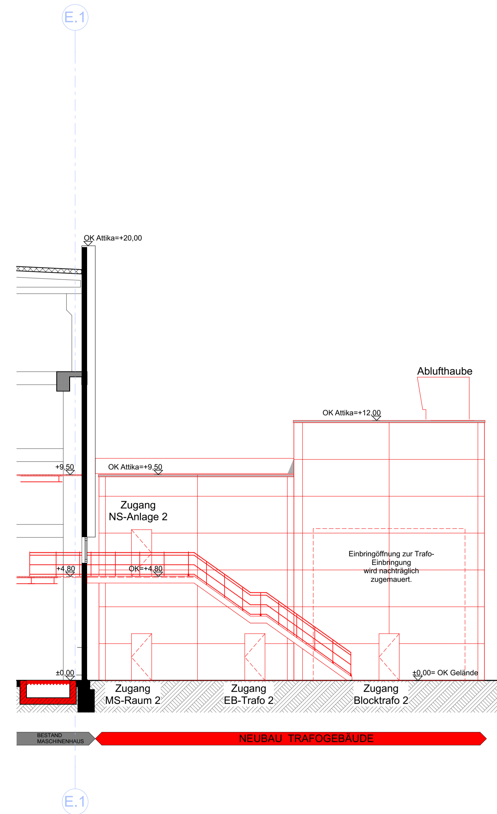
Ansicht West Trafogebäude 2
