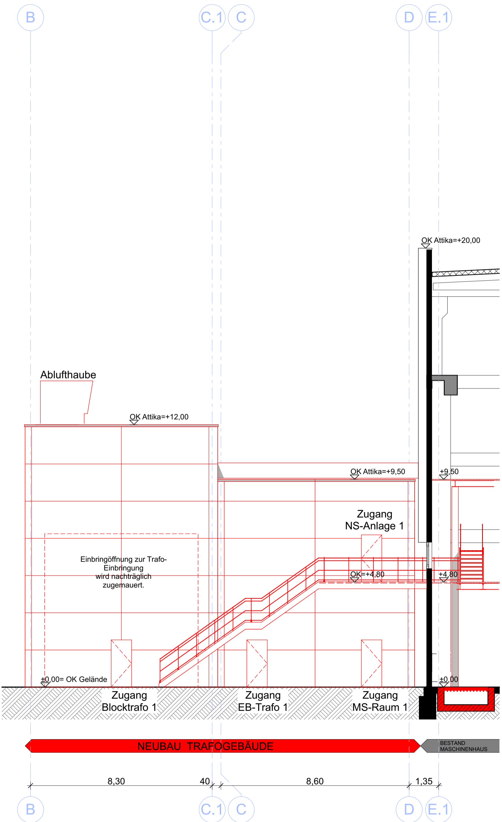
Ansicht Ost Trafogebäude 1
